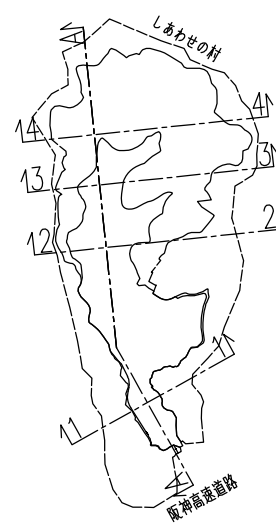
図1-3-11 2期工事土工横断図(B案)
