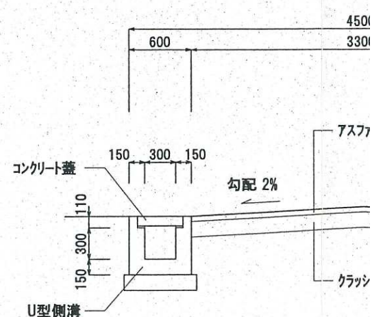
標準横断面図 (S = 1 : 50)
