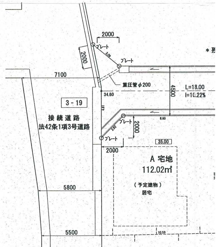
道路図 (平面図) (S = 1 : 200)
