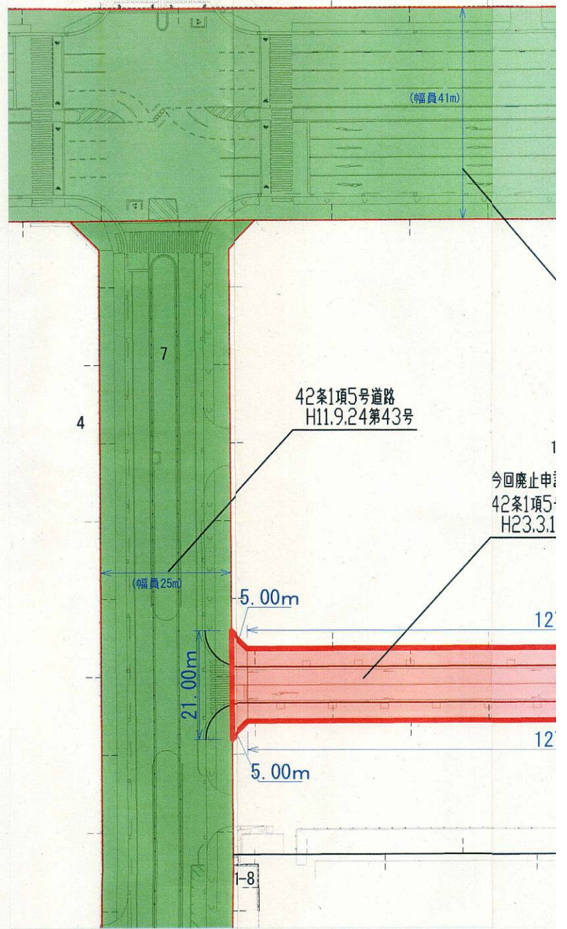
平面図 1/1,000
