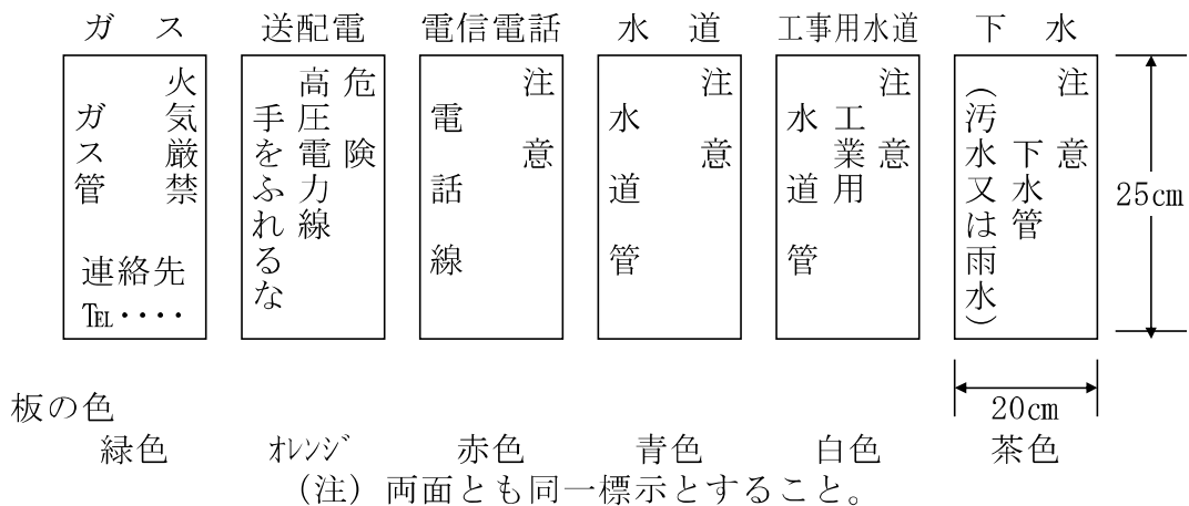
図1-2 露出する埋設物の標示板
