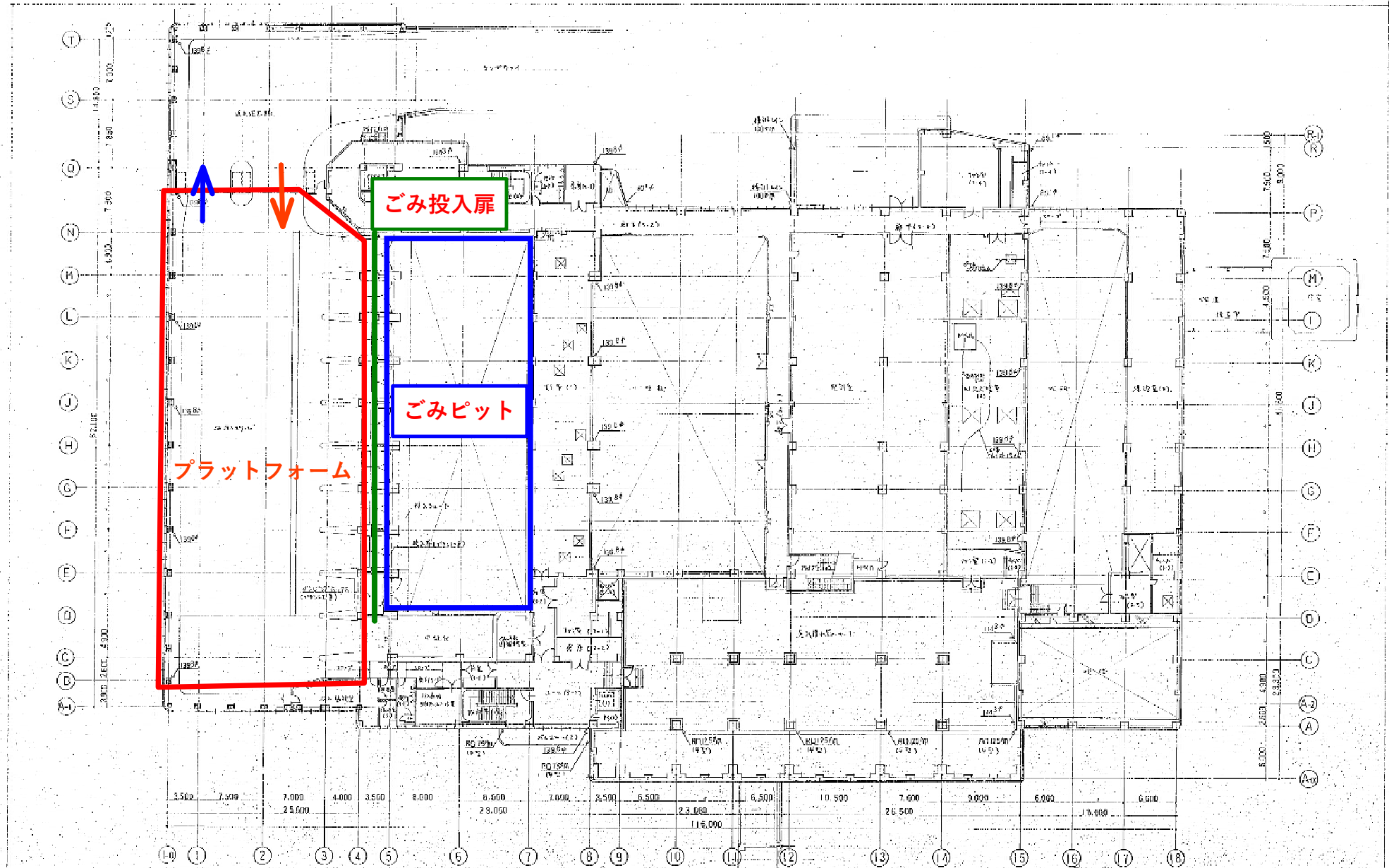
苅藻島クリーンセンター計量等業務 平面図 (工場棟3) 神戸市環境局施設課
