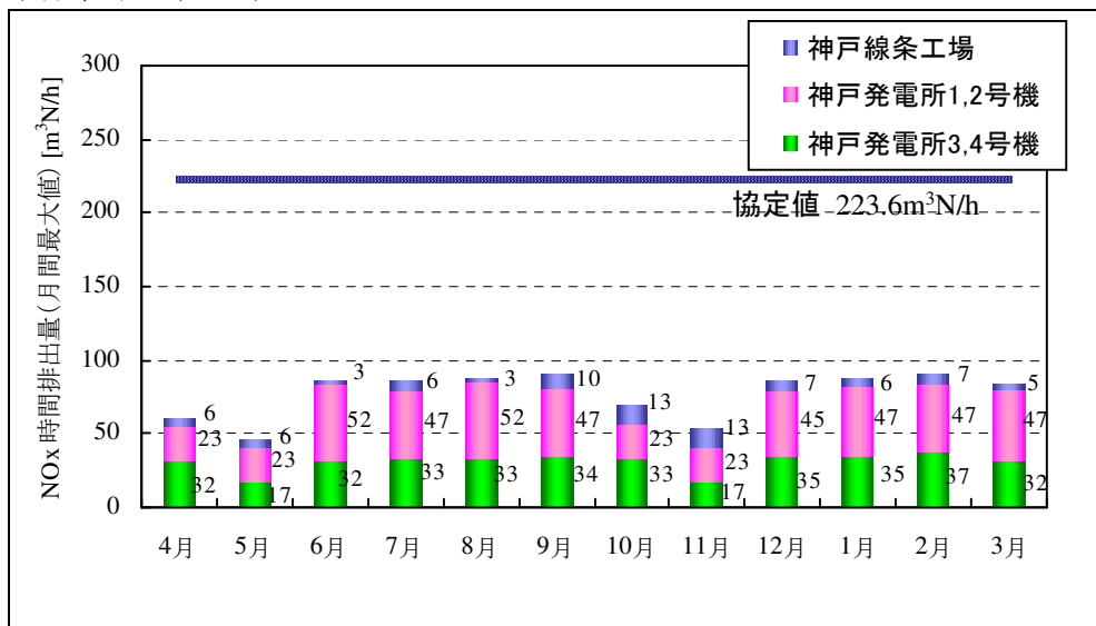
図 3-4 事業場からの NOx 時間排出量 (月間最大値)
