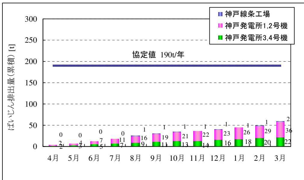
図 3-9 事業場からのばいじん排出量（累積）
