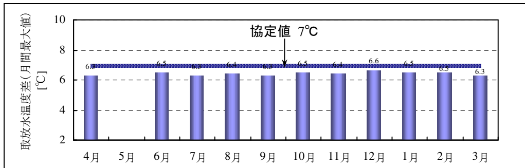
図 8-9 神戸発電所 4 号機の取放水温度差（月間最大値）
