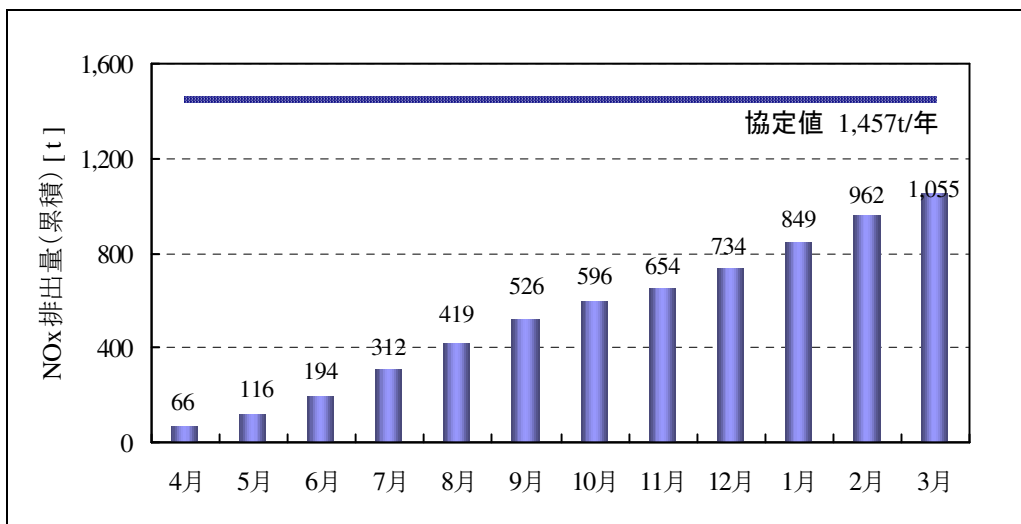
図 6-7 事業場からの NOx 排出量 (累積)
