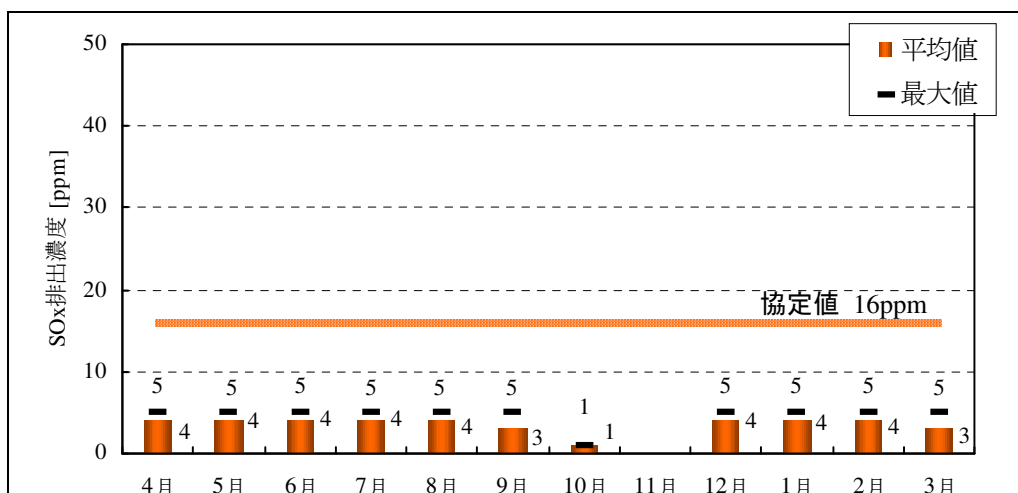
図 6-11 神戸発電所 2 号機の SOx 排出濃度
