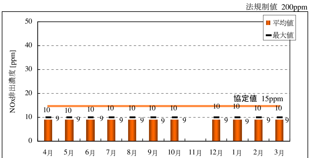
図 6-19 神戸発電所 3号機の NOx 排出濃度
