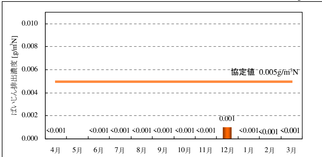
図 6-24 神戸発電所 4号機のばいじん排出濃度
