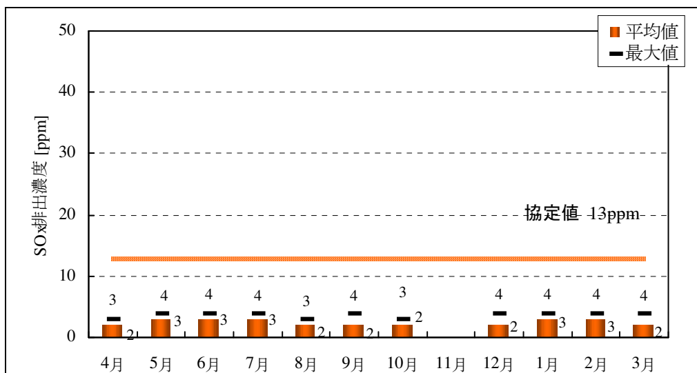
図 6-12 神戸発電所 3号機の SOx 排出濃度
