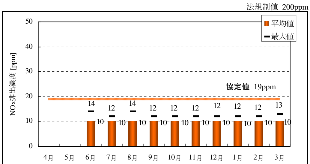
図 6-17 神戸発電所 1号機の NOx 排出濃度
