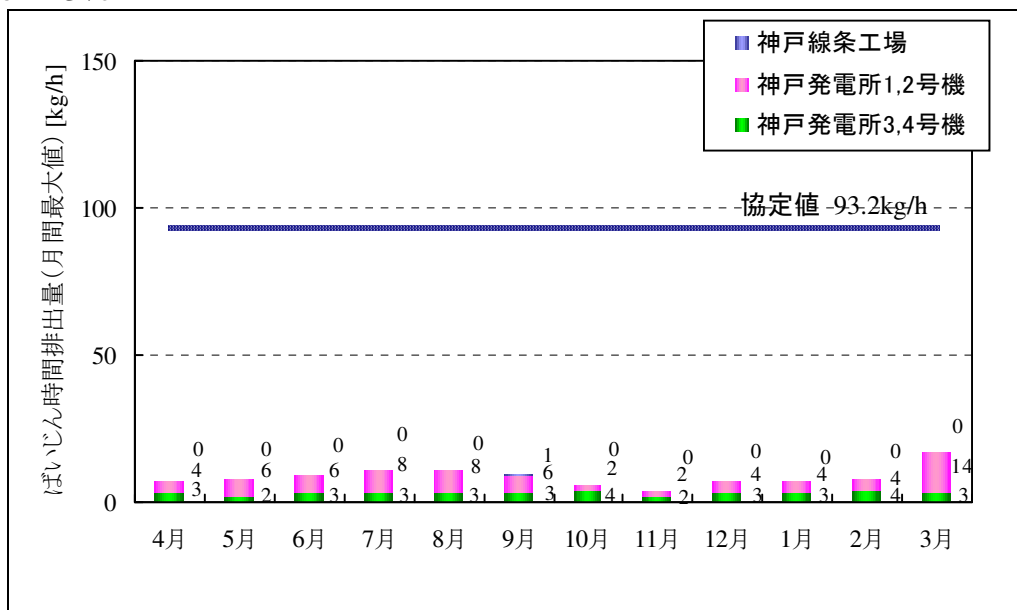
図 3-7 事業場からのばいじん時間排出量 (月間最大値)
