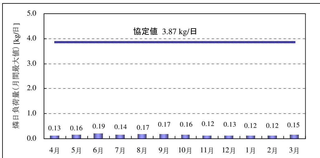
図 8-4 T-P の日負荷量 (月間最大値)
