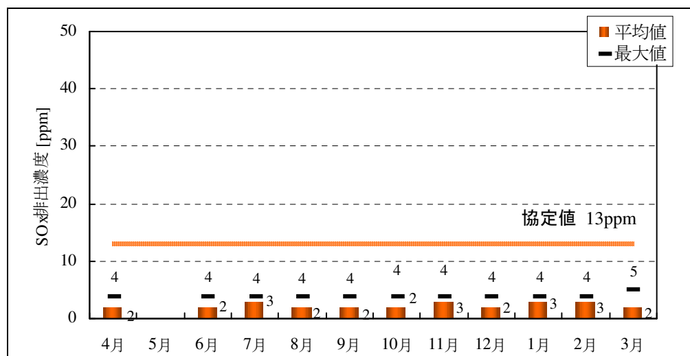
図 6-13 神戸発電所 4号機の SOx 排出濃度
