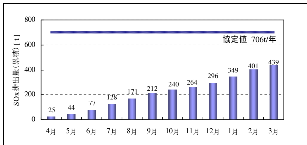
図 6-5 事業場からの SOx 排出量 (累積)
