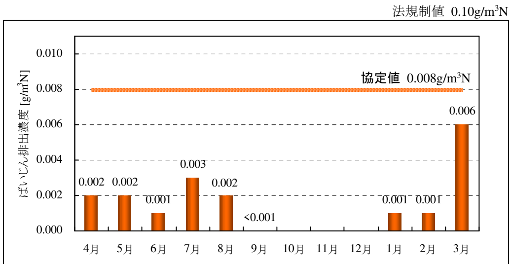
図 6-22 神戸発電所 2 号機のばいじん排出濃度
