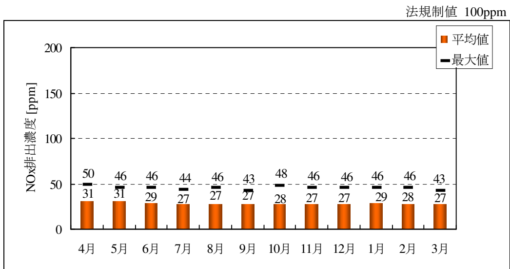
図 6-16 棒鋼工場加熱炉の NOx 排出濃度
