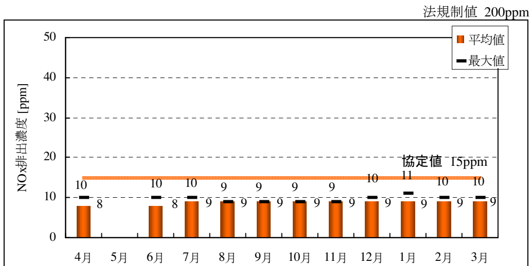
図 6-20 神戸発電所 4号機の NOx 排出濃度
