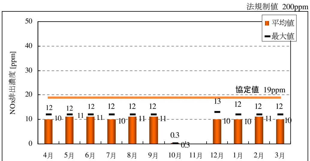
図 6-18 神戸発電所 2号機の NOx 排出濃度
