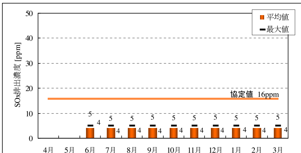
図 6-10 神戸発電所 1 号機の SOx 排出濃度
