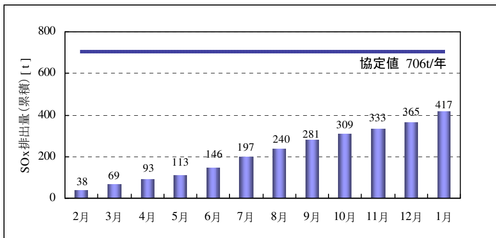
図 6-4 事業場からの SOx 排出量 (累積)
