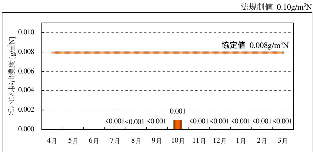
図 6-21 神戸発電所 1 号機のばいじん排出濃度
