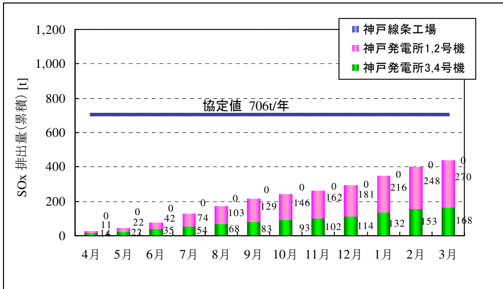
図 3-3 事業場からの SOx 排出量 (累積)
