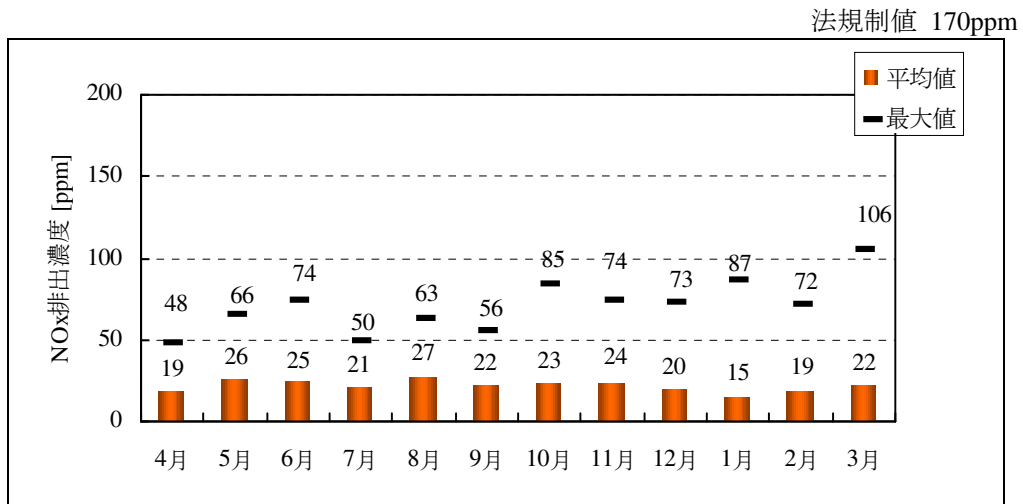
図 6-14 第 3 分塊工場均熱炉の NO x 排出濃度
