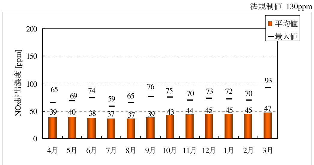
図 6-15 第 7 線材工場加熱炉の NOx 排出濃度
