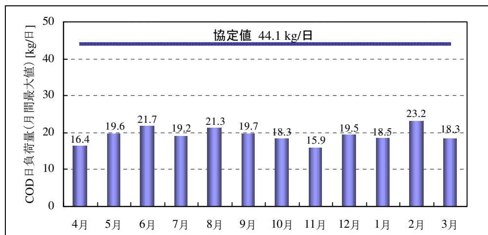
図 8-2 COD の日負荷量 (月間最大値)
