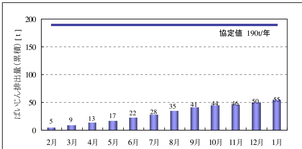
図 6-8 事業場からのばいじん排出量 (累積)
