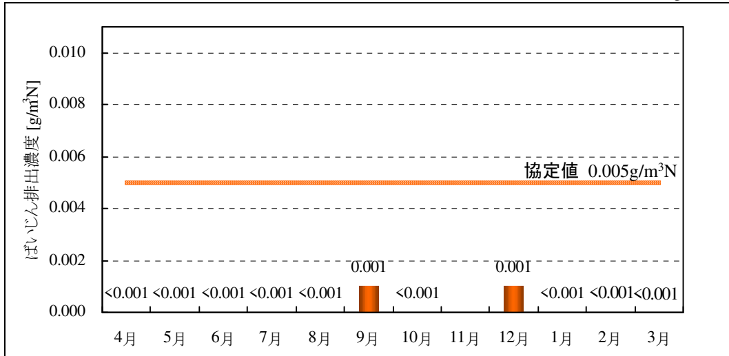
図 6-23 神戸発電所 3号機のばいじん排出濃度
